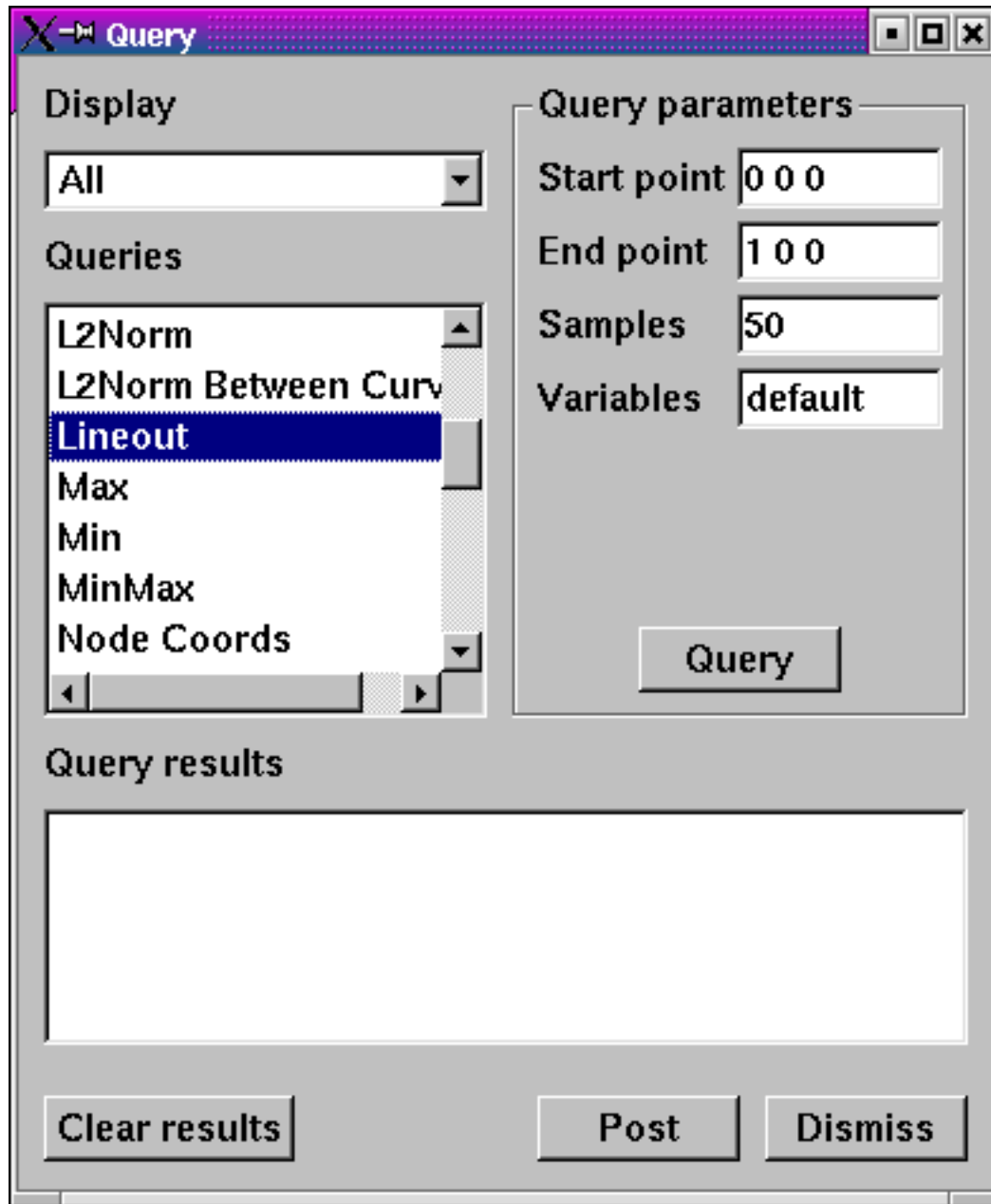
Fig. 1.201: Query window
