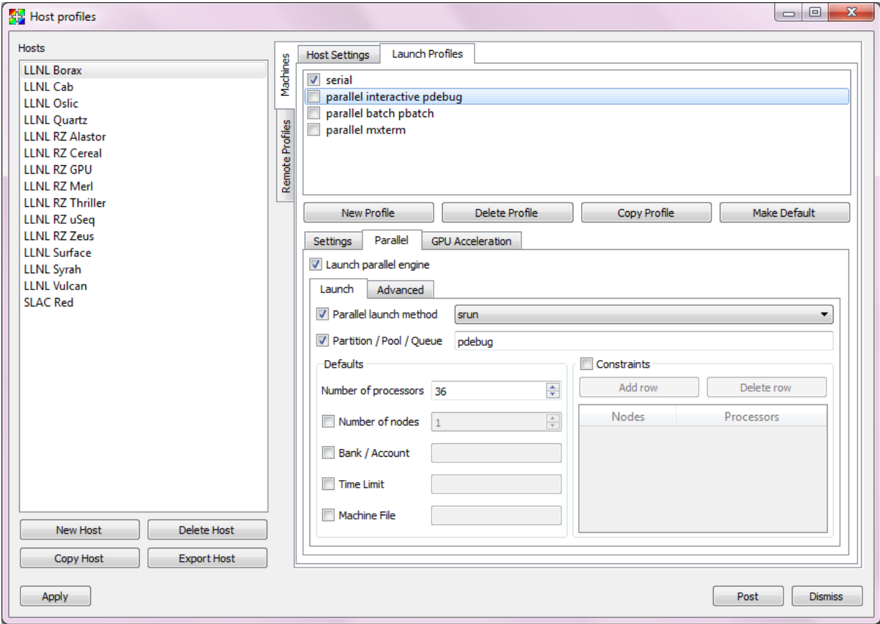
Fig. 1.308: Parallel options
