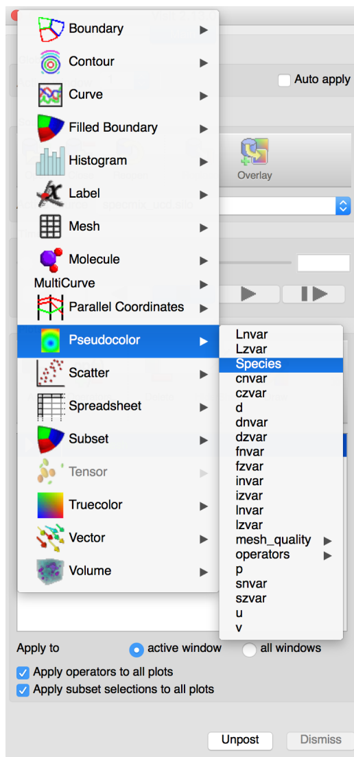
Fig. 1.194: Species variable
