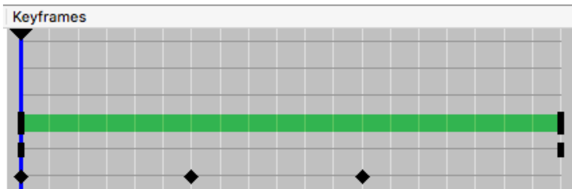
Fig. 2.303: Keyframe area
