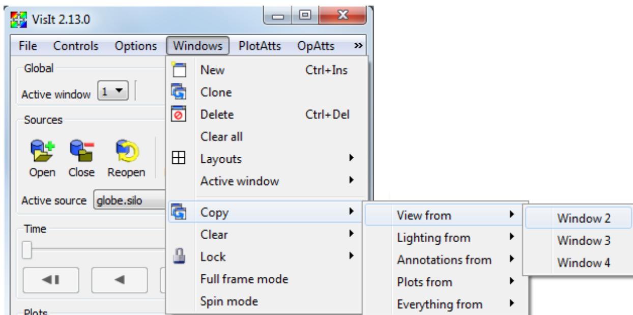
Fig. 2.184: Copy menu
