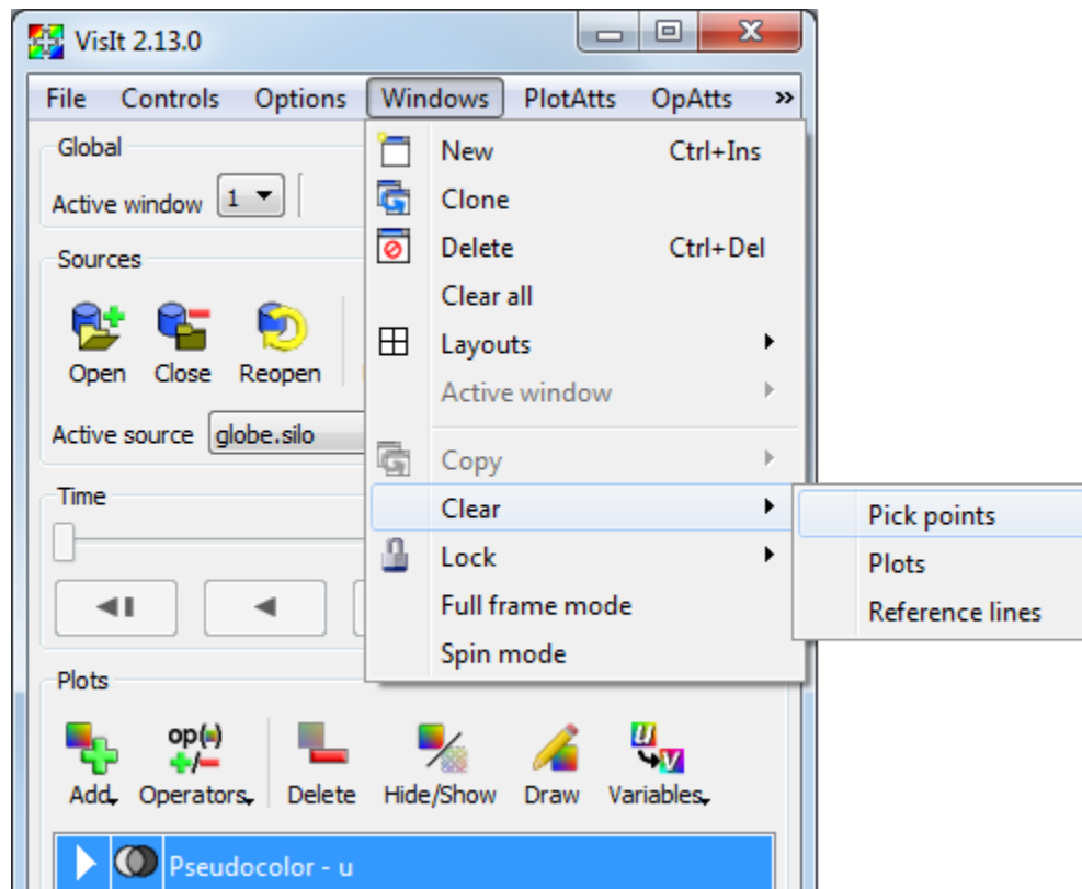
Fig. 2.182: Clear menu
