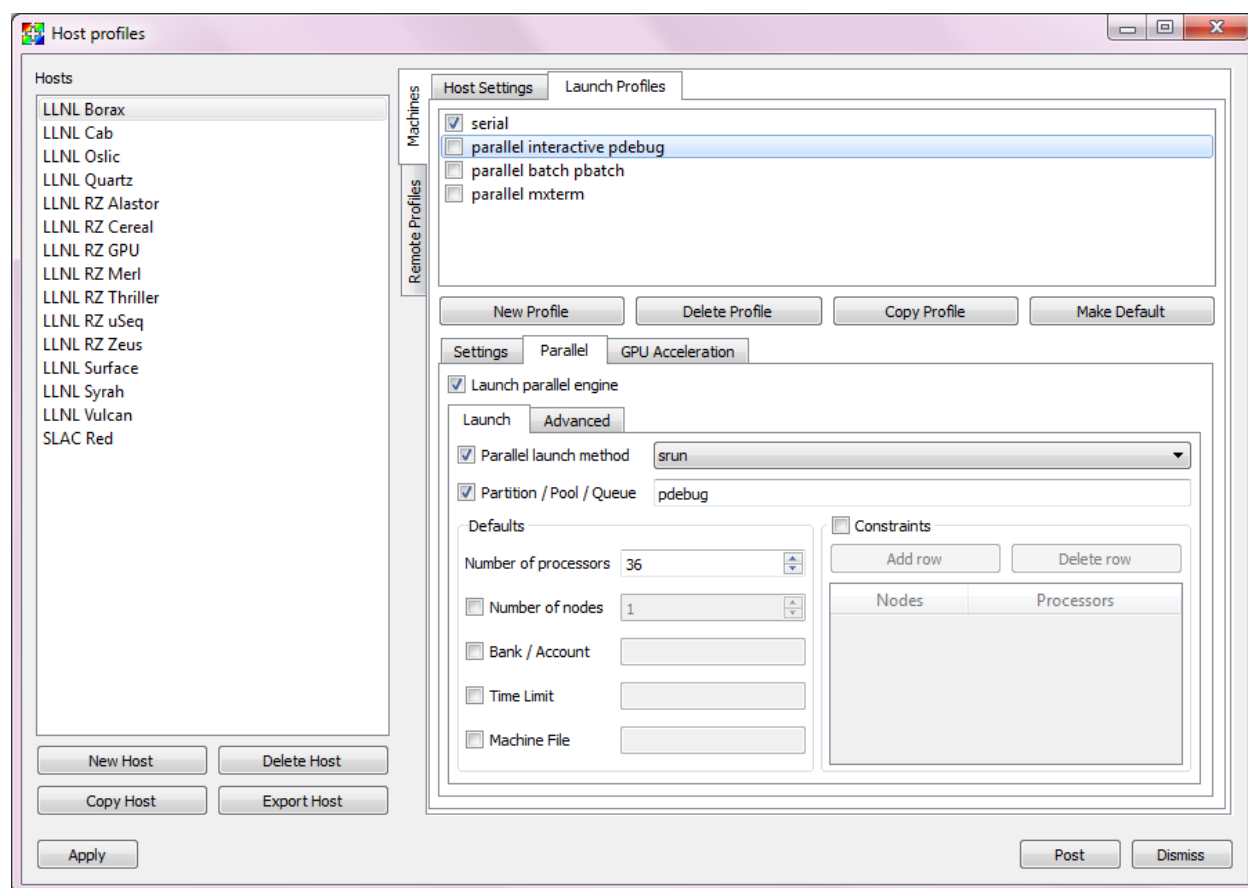
Fig. 2.341: Parallel options
