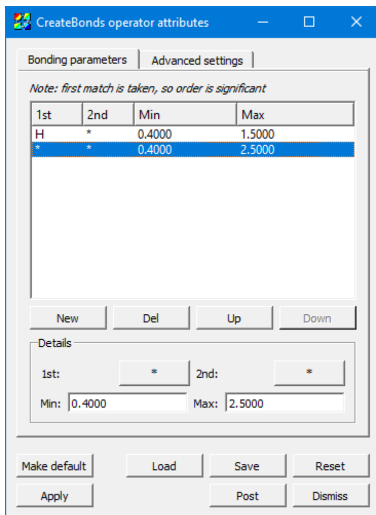
Fig. 2.100: CreateBonds bonding parameters
